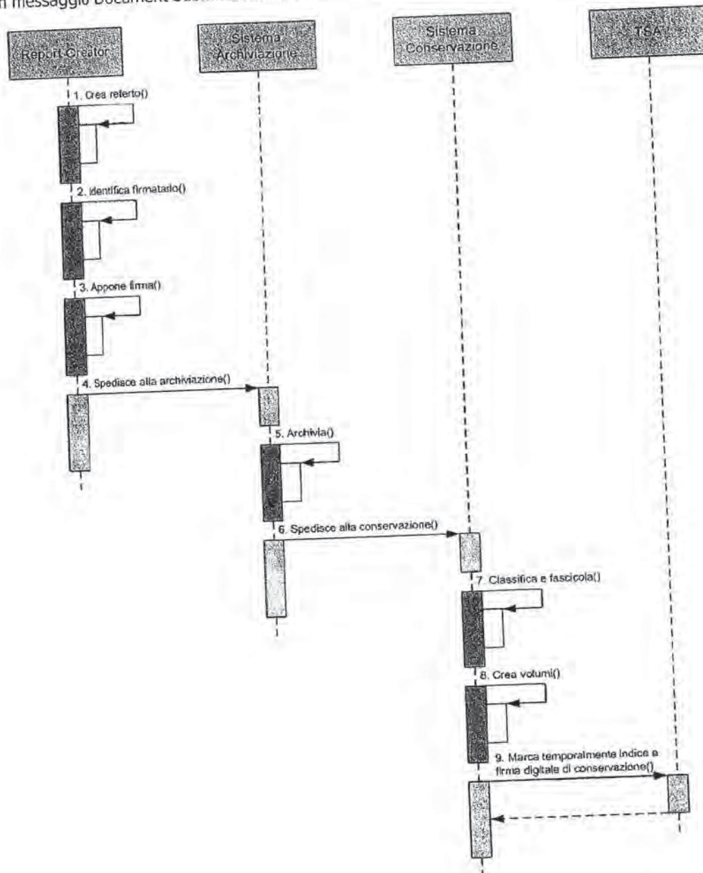
Figura 9.1: diagramma di sequenza del processo di dematerializzazione
